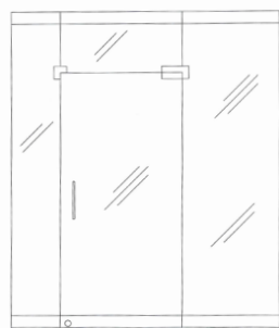
Dørparti med skinner og hjørneklumpbeslag
