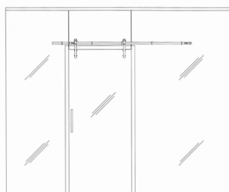
Dørparti m / U-profiler, hjørneklumpbeslag og låsekasse
